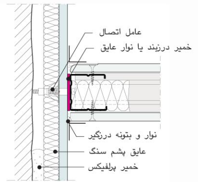
W624 - اتصال دیوار جداکننده به پوشش دیوار
