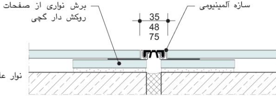
W611 - پوشش درزهای انبساط با سازه آلومینیومی
