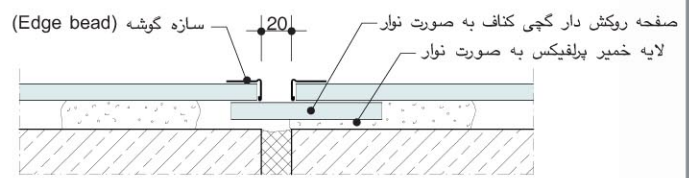
W611 - پوشش درزهای انبساط با درز نمایان
