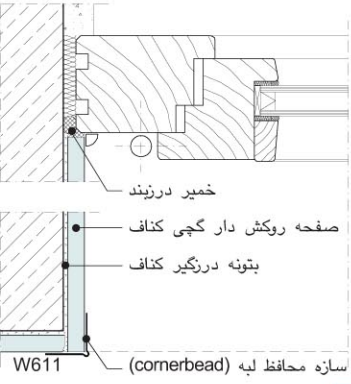
W611 - گوشه محدد
