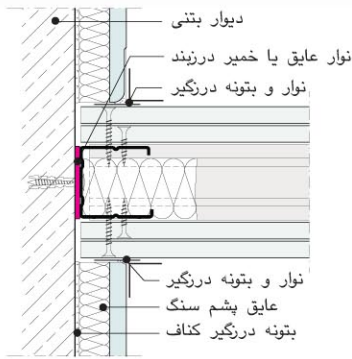
W624 - اتصال پوشش دیوار به دیوار جداکننده
