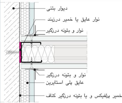
W631 - اتصال پوشش دیوار به دیوار جداکننده
