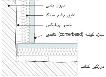
W624 - اتصال پوشش دیوار در گوشه ها
