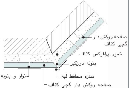
W611 - اجرای گوشه محدد
