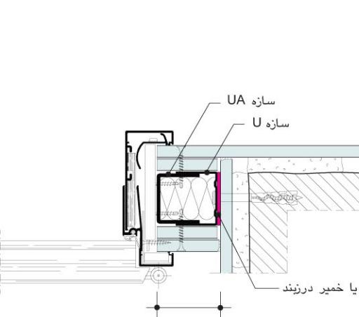
W611 - اتصال چارچوب در
